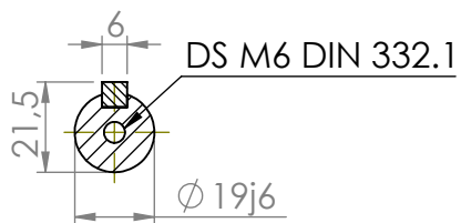
SECTION A-A SCALE 1 : 2
