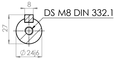
SECTION A-A SCALE 1 : 2
